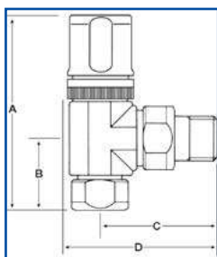
Valvola squadra / Angled valve
