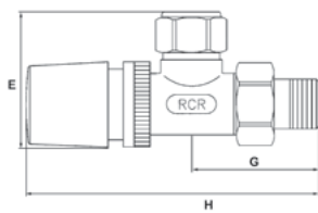
DIMENSIONI DI INGOMBRO OVERALL DIMENSIONS
